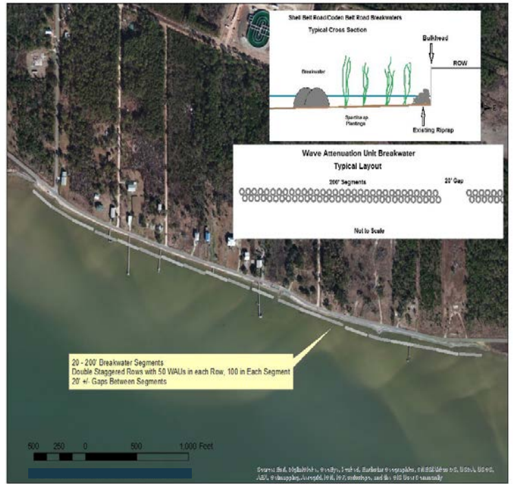
Quy hoạch dự kiến dự án Đường Bờ biển Sống Đường Shell Belt and Coden Belt.
